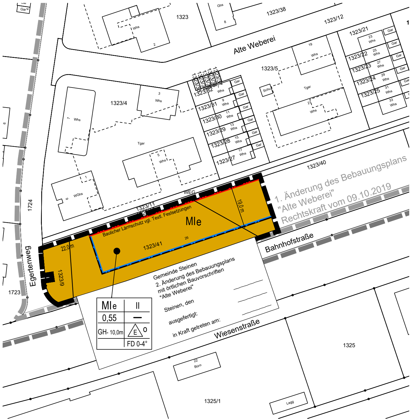
Deckblatt 2. Änderung "Alte Weberei", M 1:1.000
