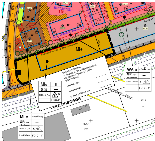
Übersicht Bebauungsplan "Alte Weberei", Fassung 1. Änderung, mit Deckblatt 2. Änderung, o.M.
